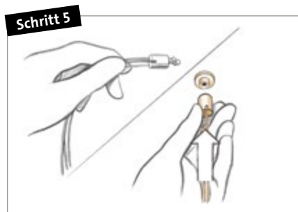
Drahtseile durch die Schraubenkappe führen und in die Deckenbefestiger eindrehen
